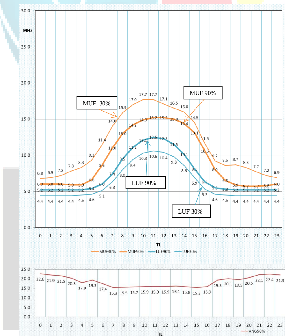
Figura 2 - Tipico andamento giornaliero delle curve rappresentative della MUF e della LUF.
