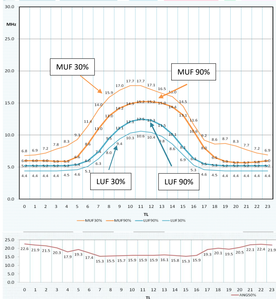
Figura 2 - Tipico andamento giornaliero delle curve rappresentative della MUF e della LUF.
